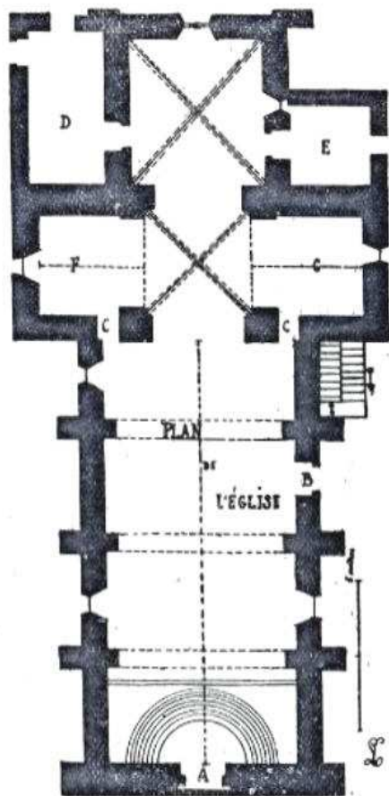
Plan de l'église Saint-Pierre à Curtil-sous-Burnand donné par Louis Chardigny (1925)
