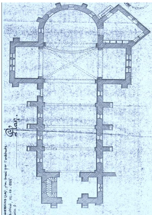
Plan de l'architecte G. Rotival (1895)
